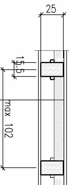
Przekrój stropu drewnianego nad parterem
